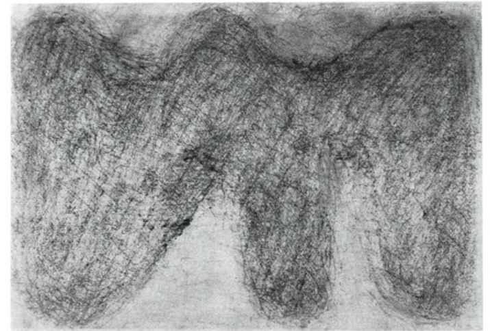
Gyűrődések, vetődések
